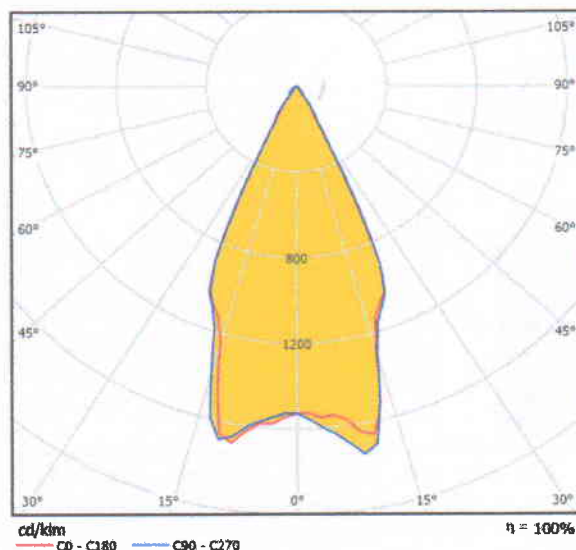
Рисунок 1 – КСС образца в поперечной (С0-С180) и продольной плоскостях (С90-С270)
